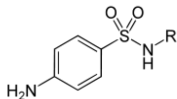
4-аминобензолсульфонамид
